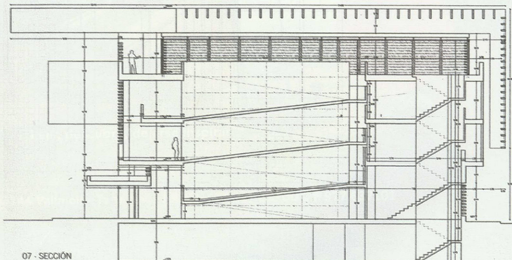
07 - SECCIÓN
